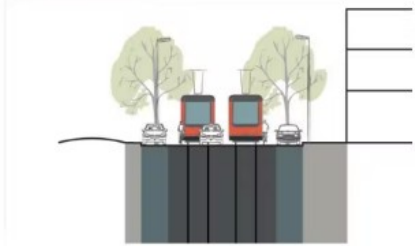
A2. Variant Fiets voor tram (2x parkeren) 1,2 - 2,0 - 8,0 - 2,0 - 3,3
