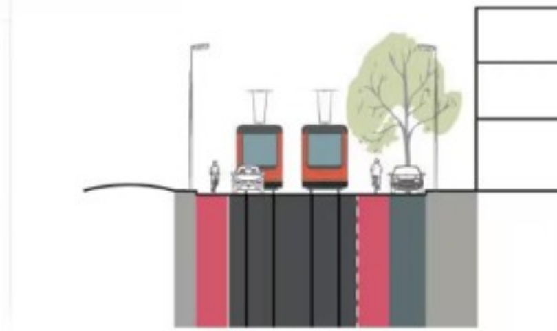
B. Variant Fietsstrook (1x parkeren) 1,2 - 10,5 - 2,0 - 2,8
